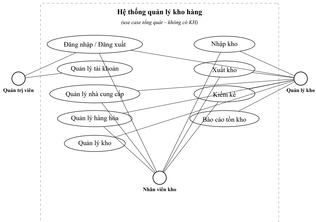
Hình 1: Sơ đồ use case tổng quát (nhóm chức năng)
